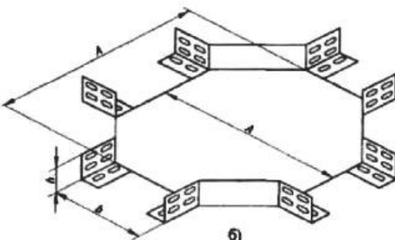
Рис 3.4.7. Лотки крестообразные
