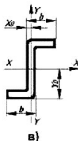
Рис. 3.6.6. Поперечное сечение профилей
