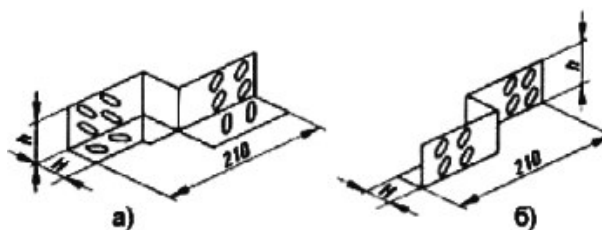
Рис. 3.4.13. Соединитель-переходник
