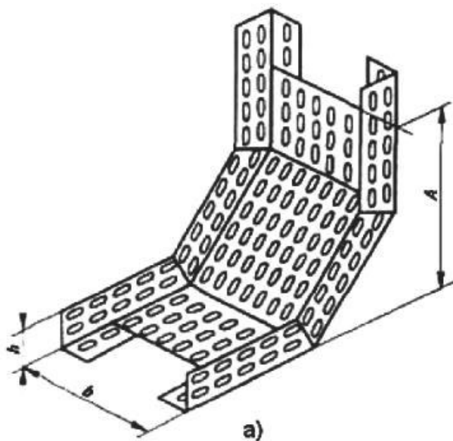
Рис 3.4.9. Лотки для поворота трассы вверх под углом 90°.
