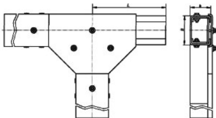
Рис.3.5.6. Короб тройниковый
