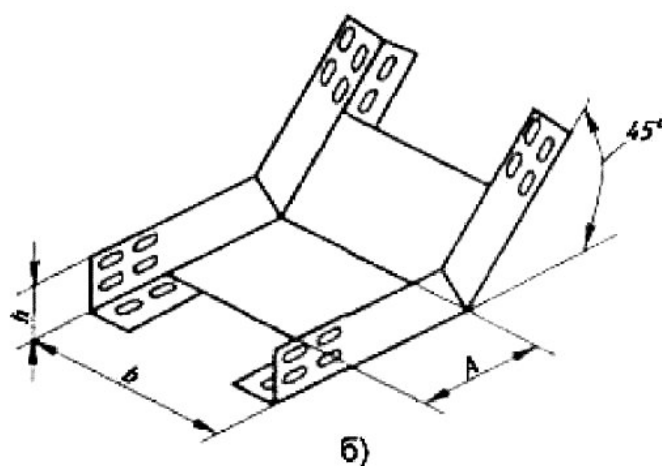
Рис 3.4.8. Лотки для поворота трассы вверх под углом 45°.
