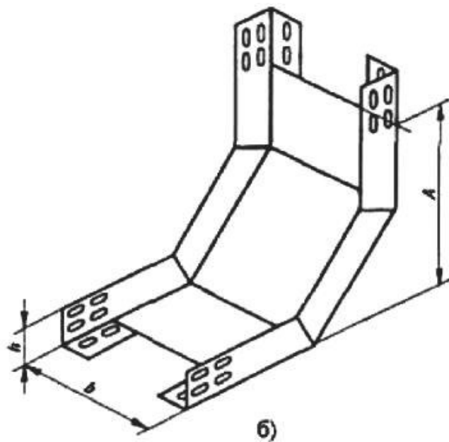
Рис 3.4.9. Лотки для поворота трассы вверх под углом 90°.
