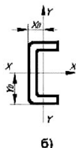
Рис. 3.6.6. Поперечное сечение профилей
