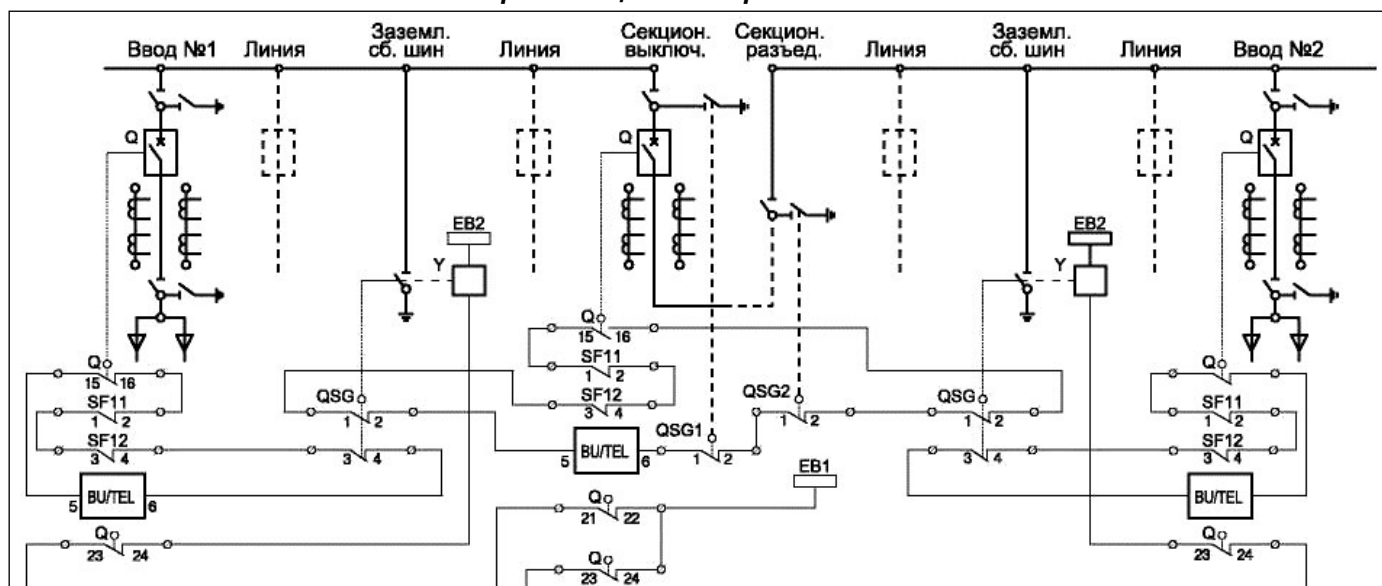
Рис. 1.2.8 Схема организации блокировок в типовом исполнении
