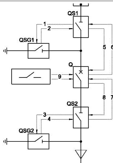
Q - выключатель вакуумный; QS1 - разъединитель шинный РВФ3-10; QSG1 - заземляющие ножи шинного разъединителя; QS2 - разъединитель линейный РВ3-10; QSG2 - заземляющие ножи линейного разъединителя
